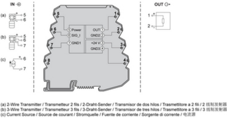
Connection Example / Exemple de raccordement / Anschlussbeispiel / Ejemplo de conexión / Esempio di collegamento / 连接示例
