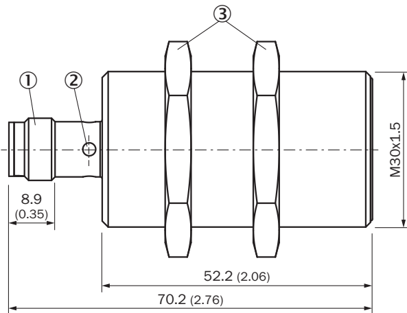
IMS30, V2A, flush
