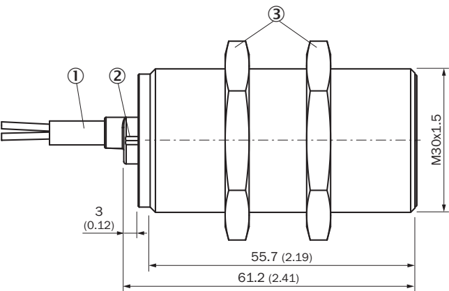
IMS30, V2A, flush
